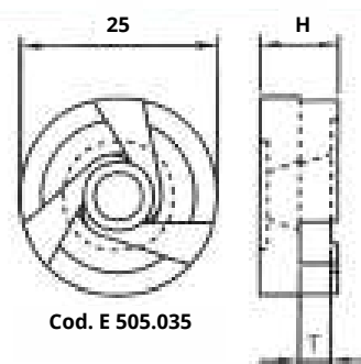
Caracola cónica 3 vías con asiento 14/19
