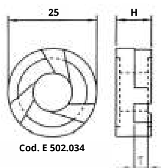
Caracola cilíndrica 3 vías con asiento para pastilla 19/19
