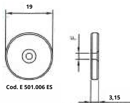
Pastilla agujereada extra especial
