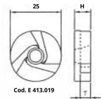
Caracola cónica 3 vías
