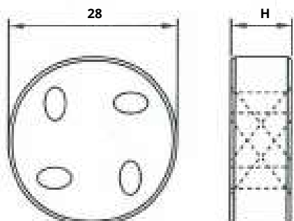
Caracola 4 vías
