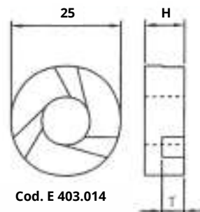
Caracola cilíndrica 3 vías
