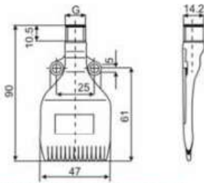
BOQUILLA SOPLADORA PEINE (AZUL) COD. 617069523
