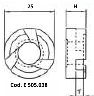
Caracola cilíndrica 3 vías con asiento 14/19
