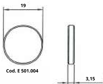
Pastilla ciega
