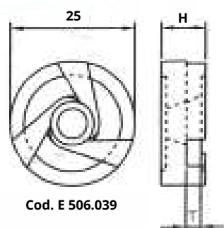
Caracola cónica 3 vías con asiento 19/19
