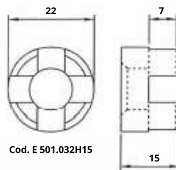
Distribuidor
